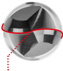
Verbesserte Kugelkopfgeometrie
